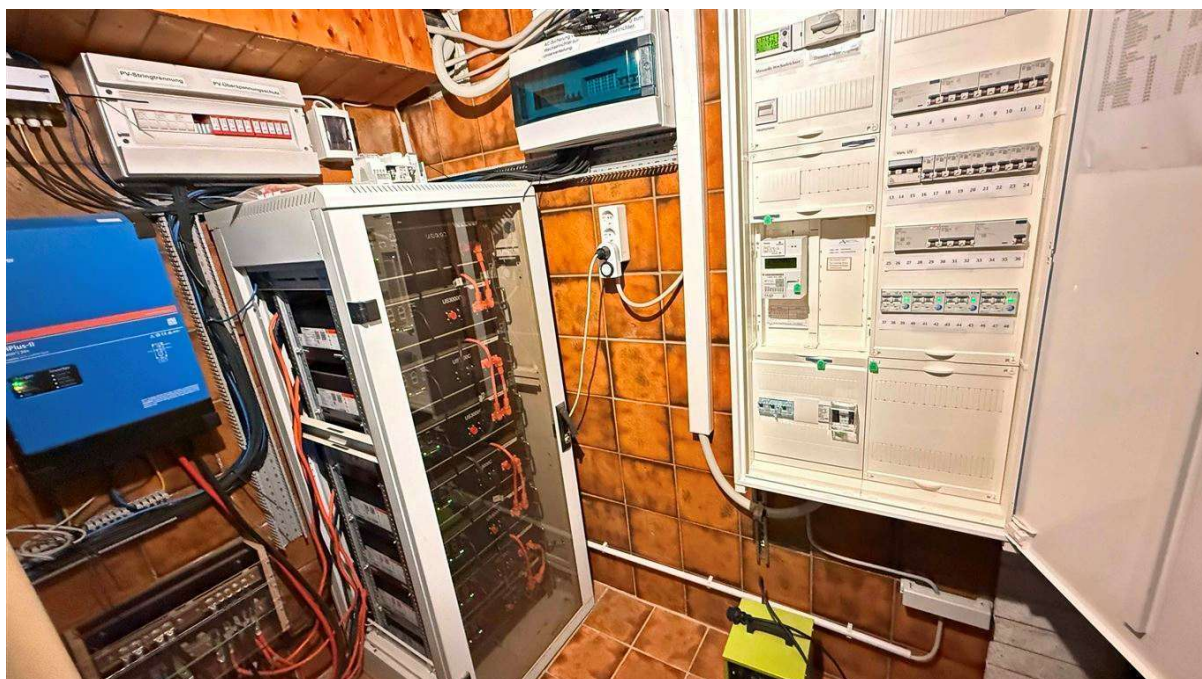
PV-Anlage 10 kWh mit Stromspeicher 24 kWh
